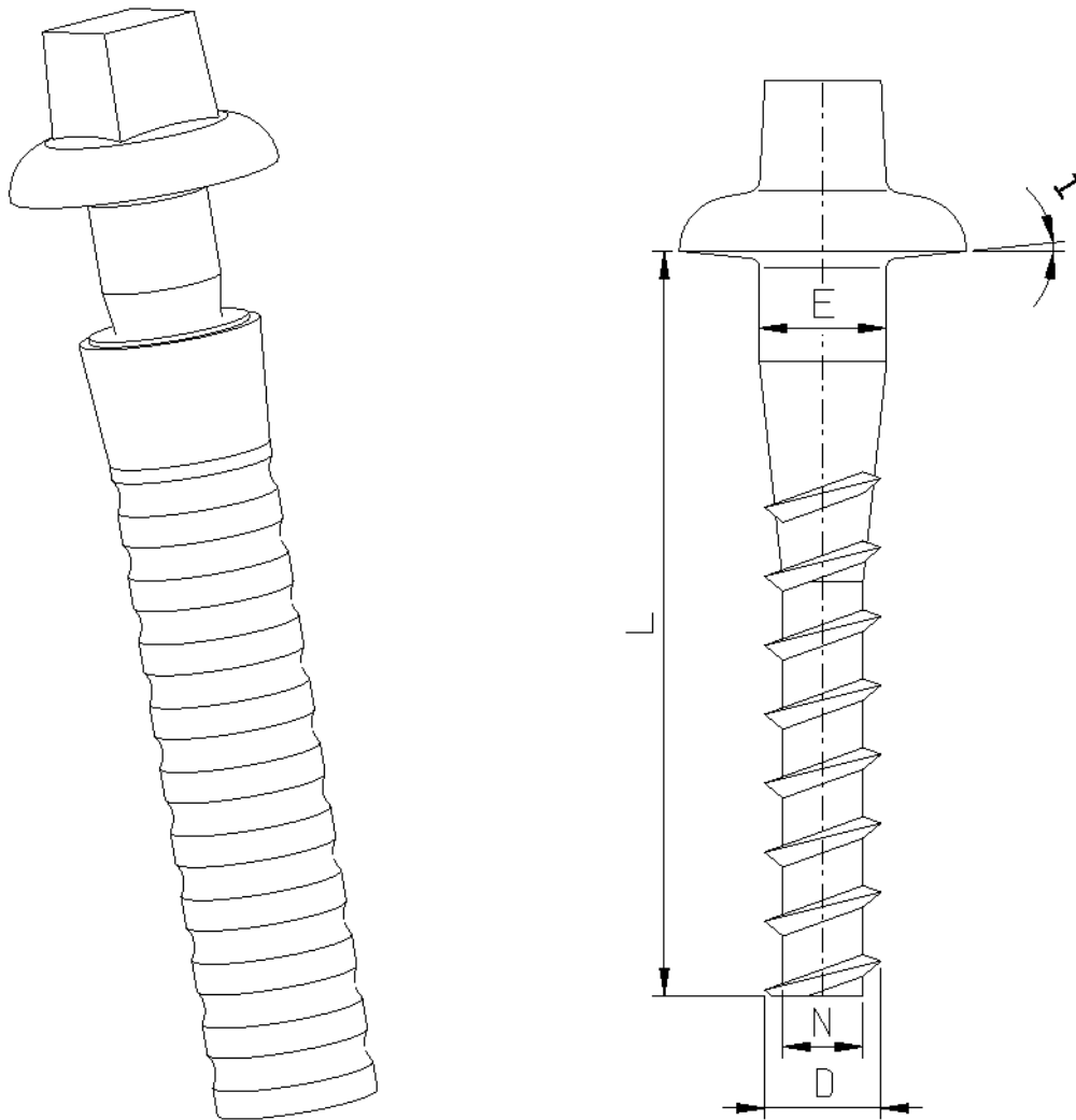
Tire-fonds suivant norme NF 50-003 – Acier qualité 4.6.
